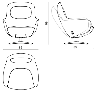
AH 7090TM low back lounge chair with lockable tilting mechanism poltrona lounge con schienale basso con meccanismo oscillante bloccabile fauteuil lounge à dossier bas avec mécanisme basculant blocable
