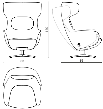
AH 9090TM low back lounge chair with lockable tilting mechanism poltrona lounge con schienale alto con meccanismo oscillante bloccabile fauteuil à dossier haut avec mécanisme basculant blocable
