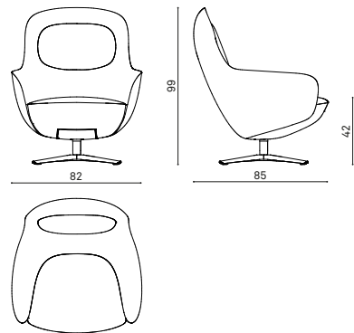
AH 7090 low back lounge chair poltrona lounge con schienale basso fauteuil lounge à dossier bas
