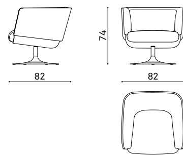
SH 7003 armchair with steel trumpet base poltrona con base a tromba in acciaio fauteuil avec base en forme de trompette en acier
