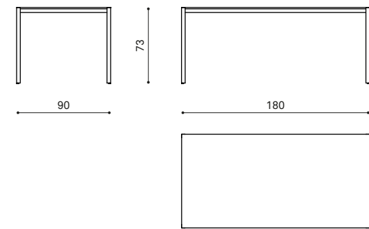
SR 18090 table 180x90x73 tavolo 180x90x73 table 180x90x73
