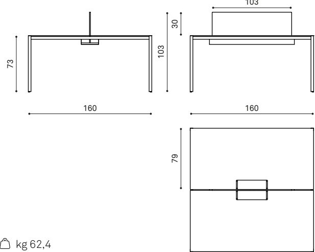
SR 160160E table with cable duct, partition panel and 2 top access 160x160x73cm tavolo con canalina passacavi, pannello divisorio e 2 top access 160x160x73cm table avec passage de câbles, panneau de séparation et 2 plateaux d'accès 160x160x73cm
