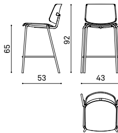
TA 6505 4 legs stool H92cm sgabello a 4 gambe H92cm tabouret à 4 pieds H92cm Upholstered Imbottito Rembourré
