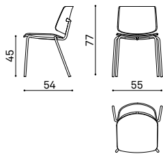
TA 1004 4 legs chair sedia a 4 gambe chaise à 4 pieds Upholstered Imbottito Rembourré
