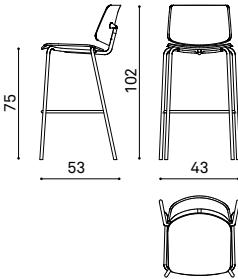
TA 7505 4 legs stool H102cm sgabello a 4 gambe H102cm tabouret à 4 pieds H102cm Upholstered Imbottito Rembourré
