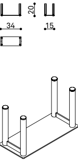
SY JJ00 junction element elemento di collegamento élément de connexion
