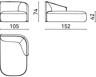
SY 1P00L/L left peninsula module modulo penisola sinistro module péninsule gauche
