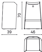
NM 200H Stool Sgabello Tabouret
