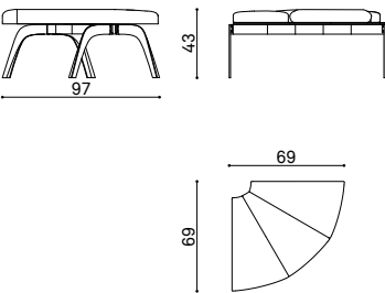
MP A000 corner element elemento angolare élément angle
