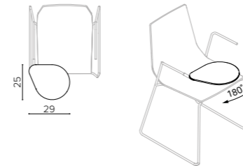
MA 10WT5 black polypropylene writing tablet only for armrest variants tavoletta scrittoio in polipropilene nero solo per varianti con bracciolo tablette d'écriture en polypropylène noir pour les variantes avec accoudoirs
