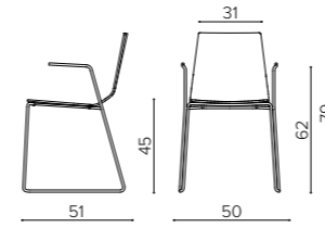
MA 1055 steel rod sled base chair with armrests sedia su slitta in tondino d'acciaio con braccioli chaise traîneau à structure en tige d'acier avec accoudoirs
