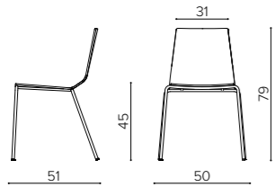
MA 100T 4 legs steel rod base chair sedia a 4 gambe in tondino d'acciaio chaise en fil d'acier à 4 pieds
