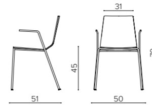
MA 104T 4 legs steel rod base chair with armrests sedia a 4 gambe in tondino d'acciaio con braccioli chaise en fil d'acier à 4 pieds avec accoudoirs
