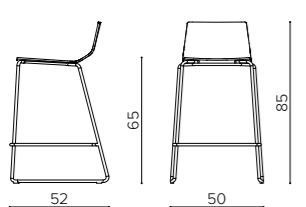
MA 6505 steel rod sled frame stool sgabello su slitta in tondino d'acciaio tabouret à structure en fil d'acier
