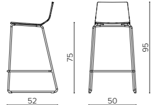
MA 7505 steel rod sled frame stool sgabello su slitta in tondino d'acciaio tabouret à structure en fil d'acier
