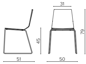
MA 1005 steel rod sled base chair sedia su slitta in tondino d'acciaio chaise traîneau à structure en fil d'acier
