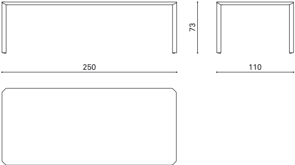
ER 250 table 250x110cm tavolo 250x110cm table 250x110cm
