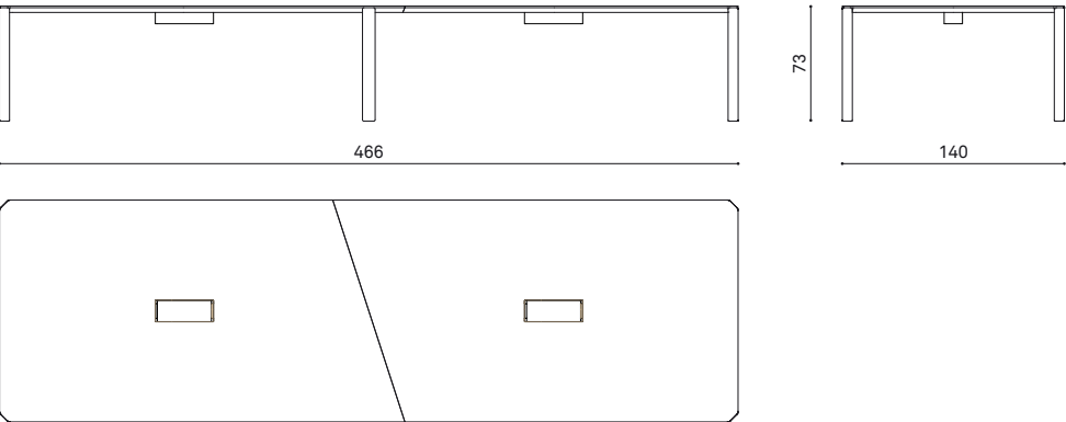
ERB 466140 table 466x140cm tavolo 466x140cm table 466x140cm
