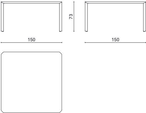
ERB 150 table 150x150cm tavolo 150x150cm table 150x150cm
