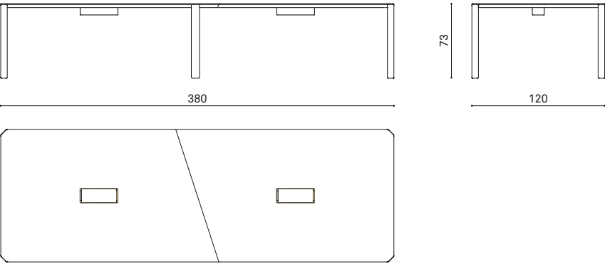
ERB 380120 table 380x120cm tavolo 380x120cm table 380x120cm
