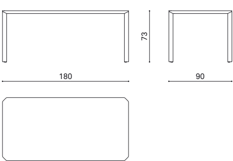
ER 180 table 180x90cm tavolo 180x90cm table 180x90cm
