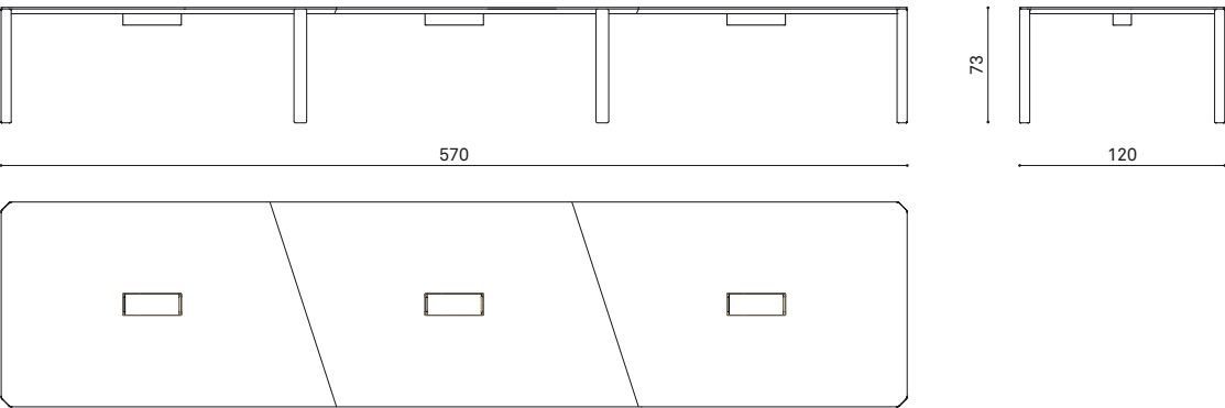
ERB 570120 table 570x120cm tavolo 570x120cm table 570x120cm
