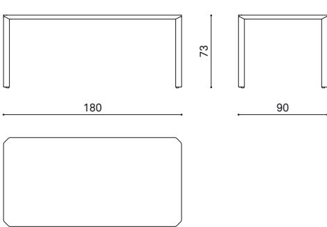
ERB 180 table 180x90cm tavolo 180x90cm table 180x90cm
