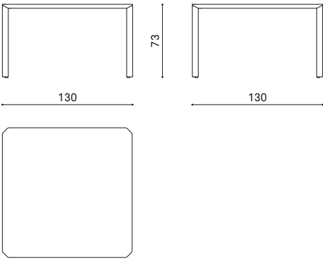
ERB 130 table 130x130cm tavolo 130x130cm table 130x130cm
