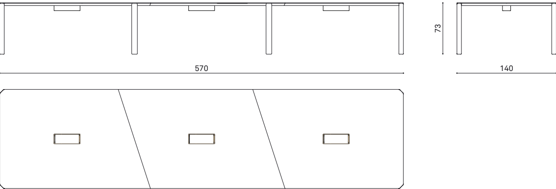
ERB 570140 table 570x140cm tavolo 570x140cm table 570x140cm
