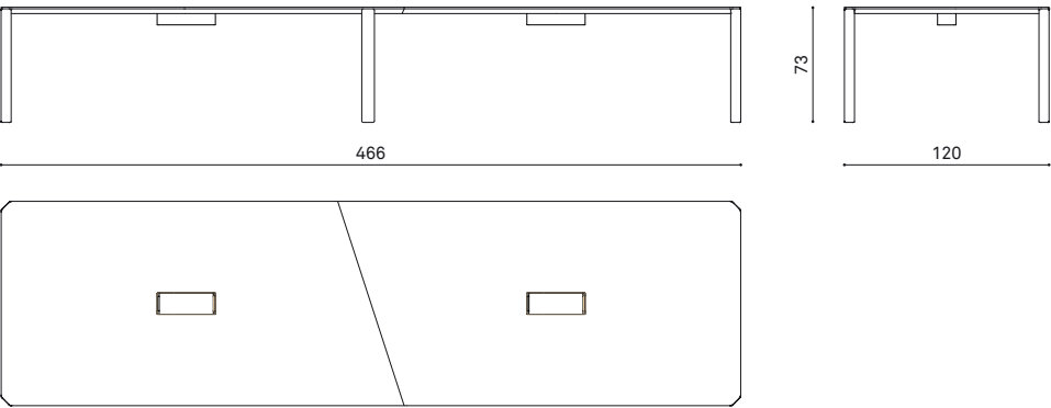
ERB 466120 table 466x120cm tavolo 466x120cm table 466x120cm
