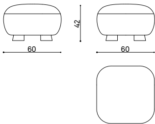
CD 60SQ OUT small square module modulo quadrato piccolo petit module carré
