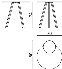
CL T70B 70cm table tavolo 70cm table 70cm
