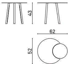
CL T30L low coffee-table tavolino basso table basse
