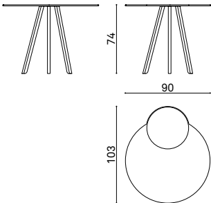
CL T90B 90cm table tavolo 90cm table 90cm
